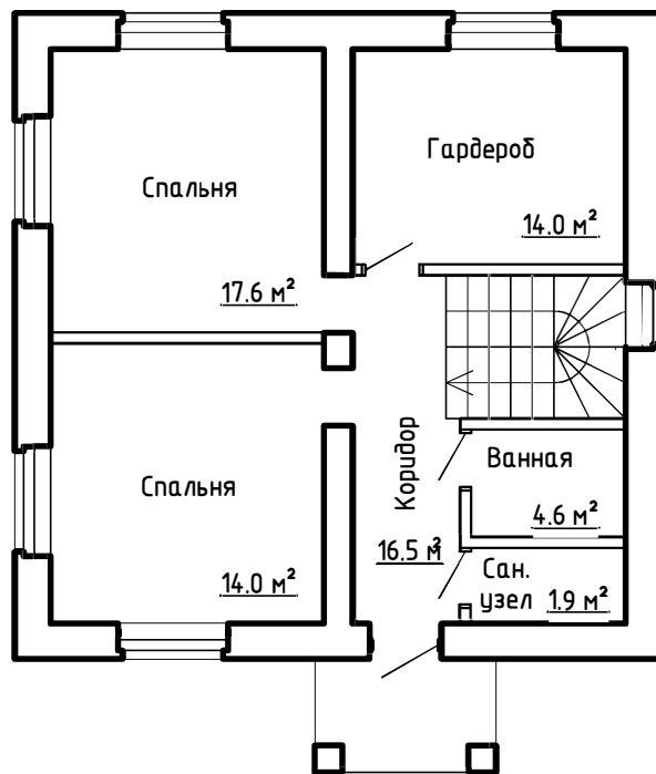
Экспликация помещений
